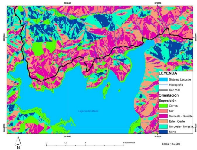
Figura 7. Cartografía de orientación. Fuente: Elaboración propia (2018).
