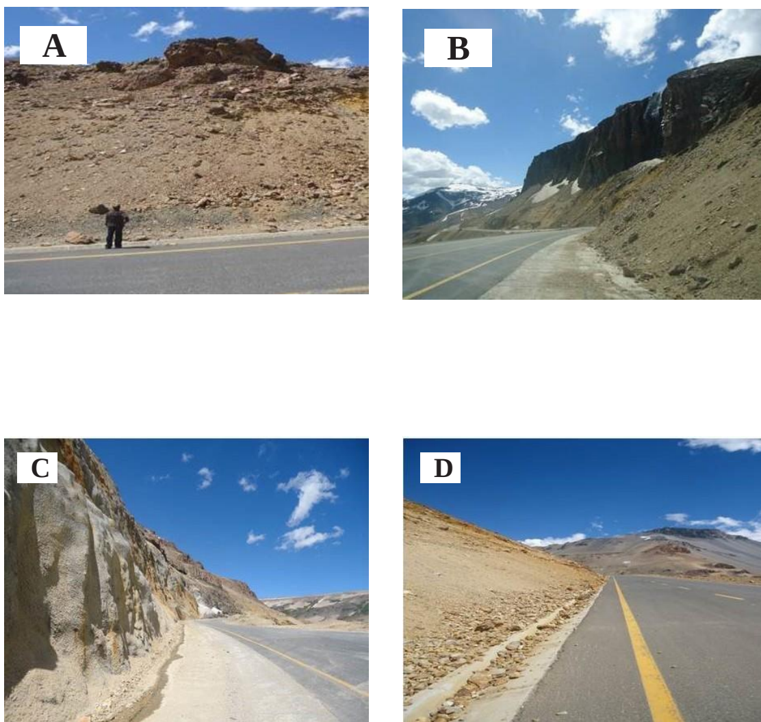
Figura 10. Deslizamientos de detritos y bloques rocosos, sector Cuesta La Zorra, Km 156, 200 al 156, 450 aprox. Punto GPS: Datum WGS 84; N 6.014.827-E 372.646 (figura 11). Macizo rocoso con alta meteorización y pendiente muy alta cercana a ruta. A) Deslizamientos de bloques rocosos de diferentes tamaños y pequeños desprendimientos de rocas. B) Vista de talud que presenta alta pendiente con deslizamientos de material. C) Talud con obras de mitigación que presentan oxidación en algunas áreas con meteorización física importante. D) Talud con gran cantidad de material cercano a camino. Fuente: Dirección de Planeamiento (DIRPLAN) (2014).
