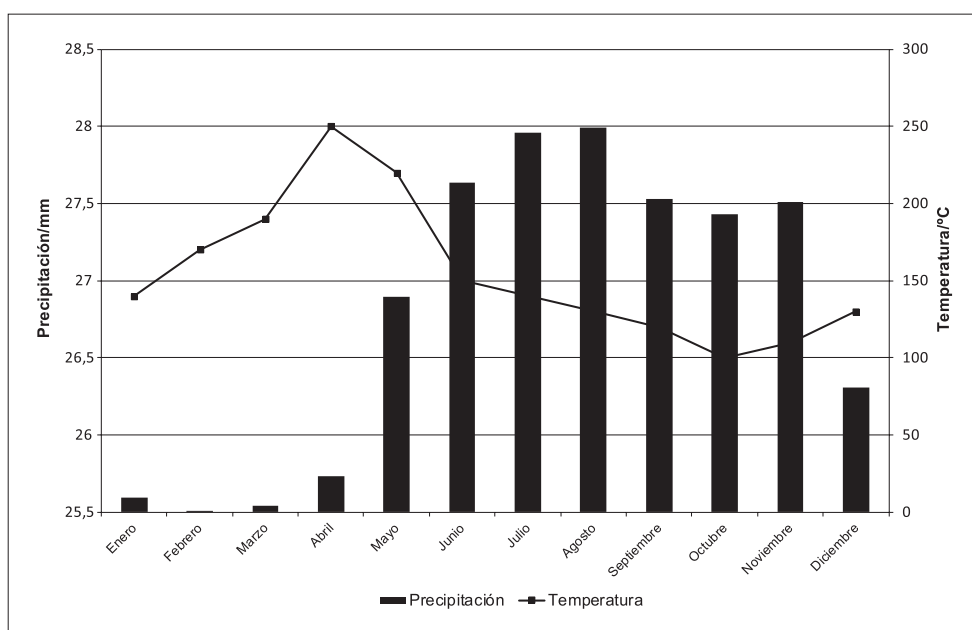
Fig. 3. Climograma de la estación meteorológica Pedasí. Años 1967 – 2013.
