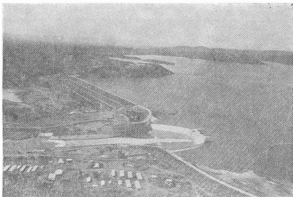
Fig 8. Presa Miguel Hidalgo sobre el río Fuerte en el Estado de Sinaloa para generar 60.000 kW. y recuperar 64.000 hectáreas de tierras ensalzadas.
