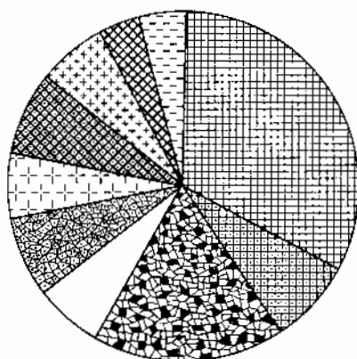
BASALTOS
