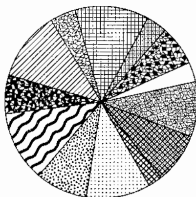
ANDESITAS PORFÍRICAS
