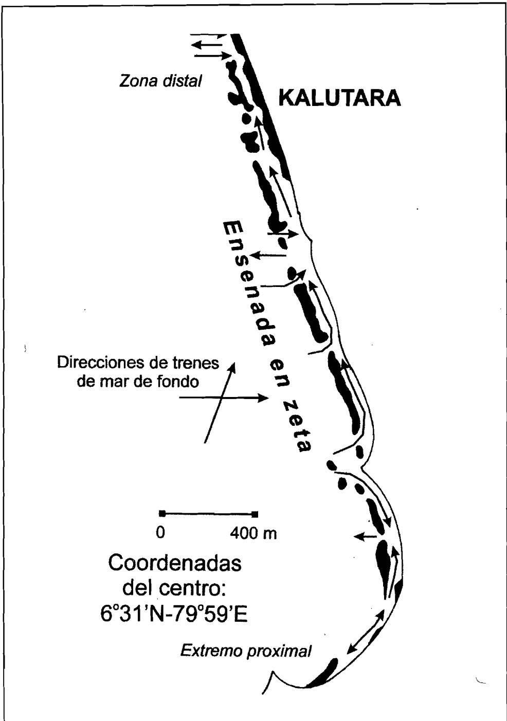
Fig. 5. Estados de zona de rompiente pre-tsunami. Efecto de ensenada, desde zona proximal (playa reflectiva) a distal (playa y barra rítmicas).
