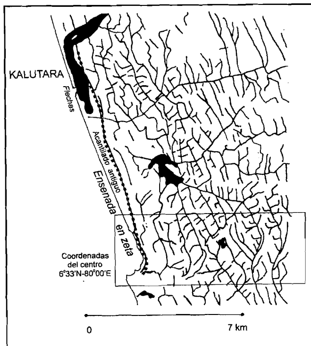
Fig. 3. Patrón de drenaje costero en enrejado direccional, indicando la influencia de las bandas de gneiss charnockítico en la línea de costa. El rectángulo muestra donde la curvatura de banda es similar a la mayor curvatura de la ensenada en zeta.
