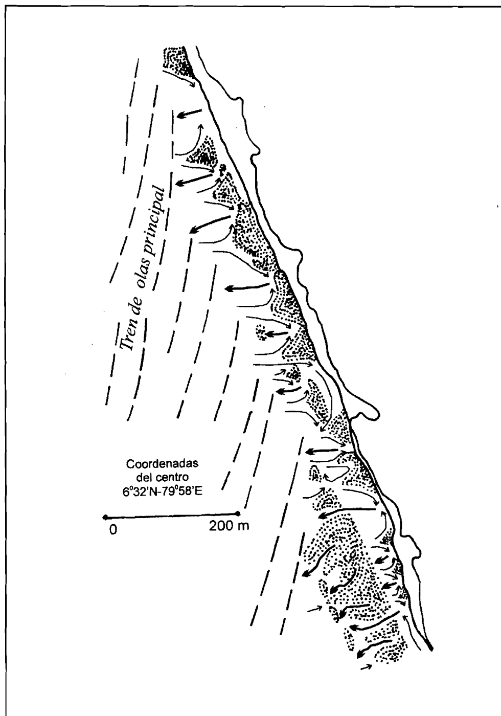
Fig. 4. Kalutara: Estado de zona de rompiente pre-tsunami, tipo barra (con trama de puntos) y surco transversal (flechas gruesas).
