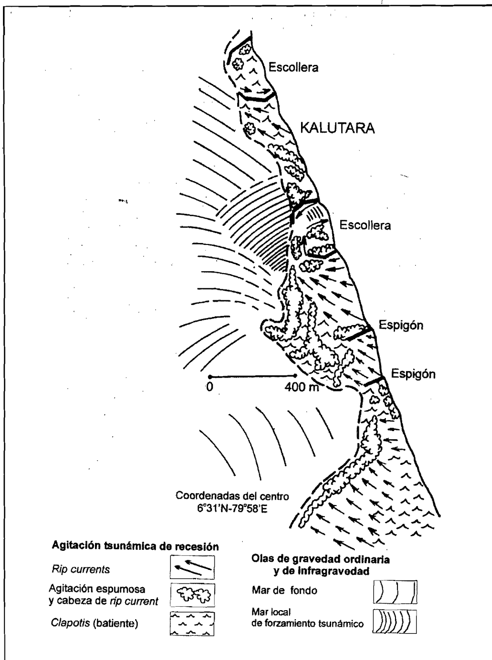
Fig. 8. Agitación tsunámica de recesión vs. olas de gravedad ordinaria y de infra-gravedad (26.12.04). El límite entre ellas es indicado mediante línea segmentada. Las líneas negras anchas señalan los espigones y escolleras.
