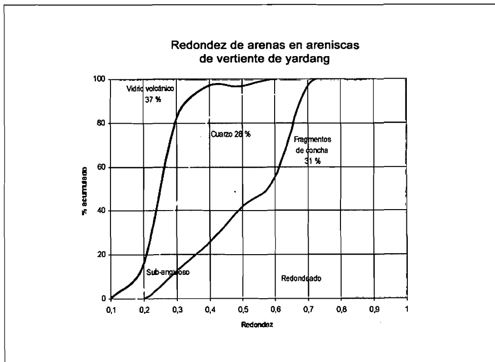
Fig. 11. Mar de Dunas Bajo Norte: arenisca de yardang .
