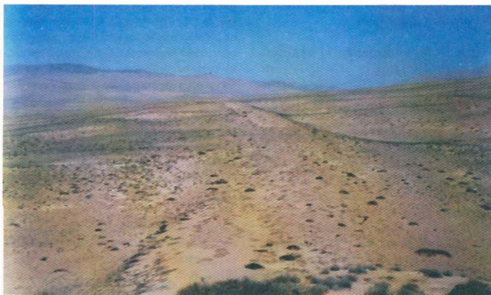
Fig. 8. Mar de Dunas Bajo Norte. Cinturón transverso-transgresivo pulso 3 recubierto por sistema lineal longitudinal pulso 4. Ambos sistemas son vegetacionados e inactivos. Fug. 8. Northern Low Sea of Sand. Transverse-transgressive belt, pulse 3 overlayed by longitudinal linear system of pulse 4. Both systems are vegetated and inactive.
