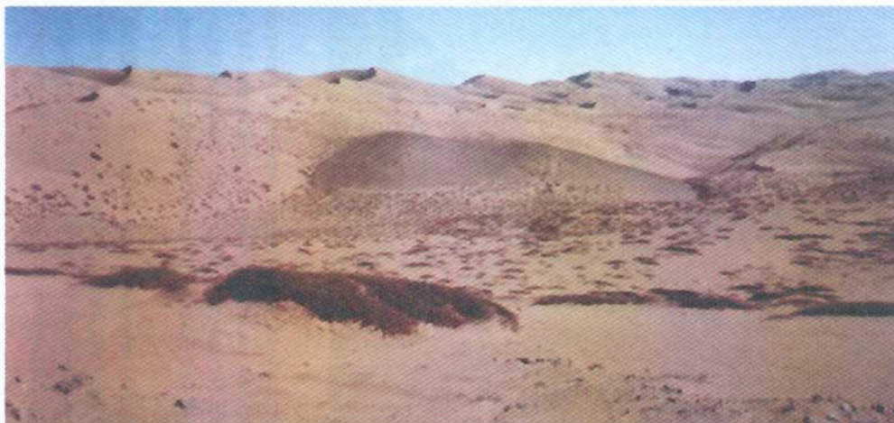
Fig. 17. Mar de Dunas Alto Norte. Detalle del aklé típico de parabólicas inactivas en primer plano (pulso 2), con vegetación esteparia baja. Al fondo, aklé activo barjánico y parabólico en la parte alta (pulso 5), con vertientes de precipitación y algunas reversas (Fig. 16).
