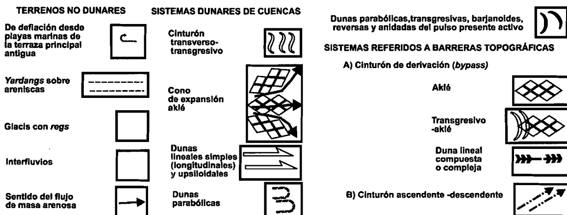
Fig. 2. Mapa geomorfológico general de los ergs de Atacama.
