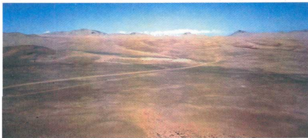
Fig. 21. Mar de Dunas Bajo Sur. Relaciones aloestigráficas entre pulsos 1, 2 y 3. Al fondo e izquierda, dunas lineales longitudinales recubriendo al aklé del pulso 1. Al frente y derecha, cinturón transgresivo- aklé recubriendo a dunas lineales.
