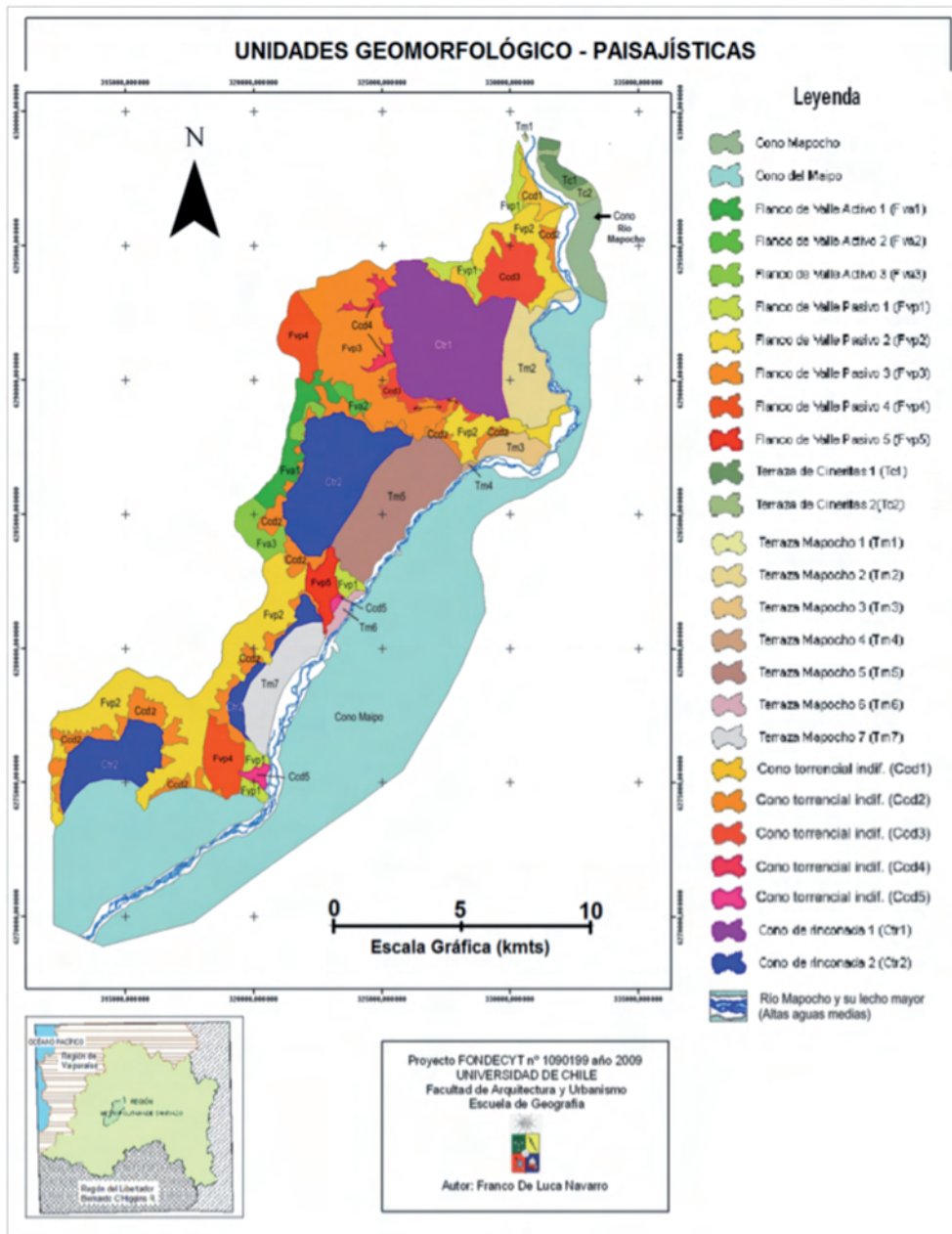
Fig. 3. Unidades Geomorfológico-Paisajísticas
